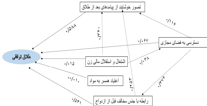
شکل ۱: تحلیل مسیر
